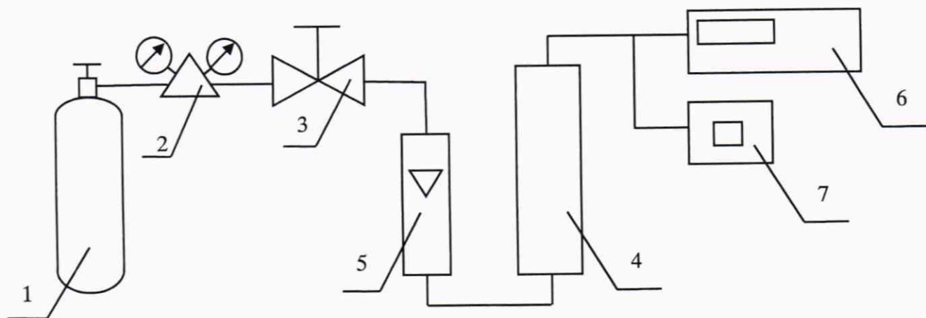
Рисунок В.2 – схема подачи ПГС из баллонов под давлением на вход аналитической части КТО – 600
