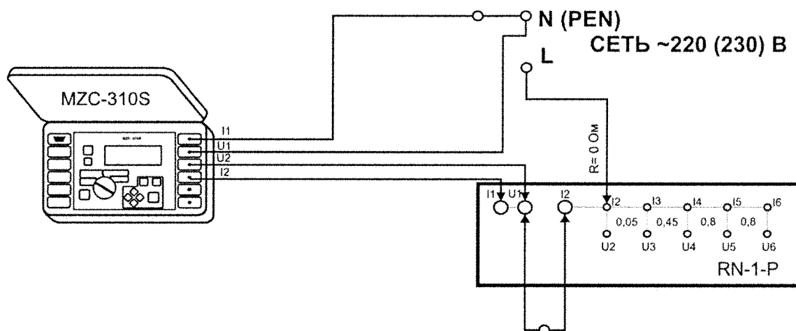
Рисунок 4 – Структурная схема определения абсолютной погрешности измерения полного сопротивления цепи 4-х проводным методом ,
