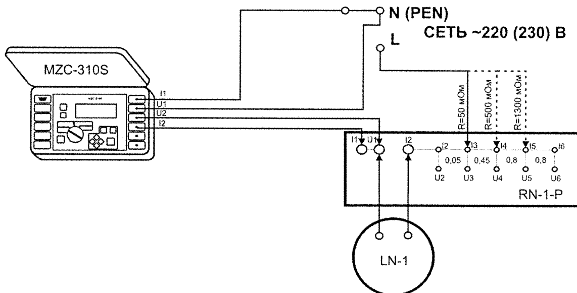
Рисунок 5 – Структурная схема определения абсолютной погрешности измерения полного сопротивления цепи 4-х проводным методом , где MZC-310S – поверяемый измеритель; RN-1-P – мера сопротивлений петли короткого замыкания.
