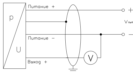
3-х пров. (вых. сигнал - напряжение)
