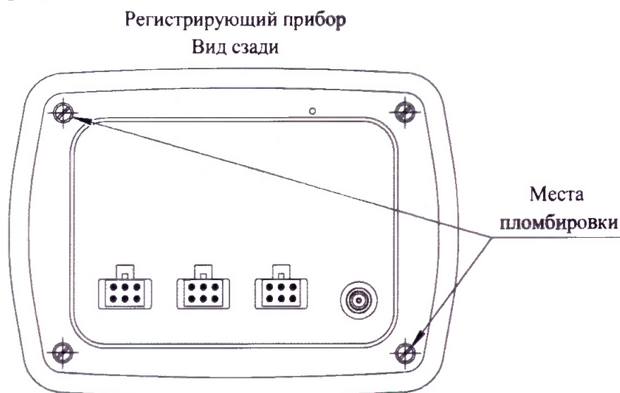
Рисунок 1 - Места пломбировки
