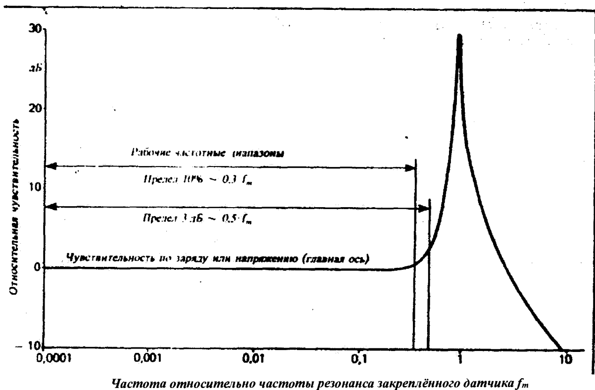
Рисунок - 1 Кривая амплитудно-частотной характеристики (АЧХ) датчика
