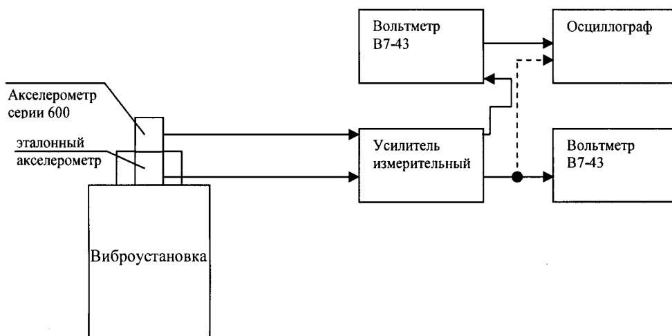
Рисунок 1 – Схема подключения акселерометра при проведении поверки
