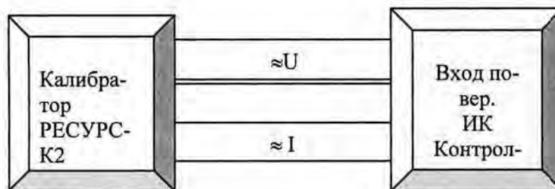
Рисунок 5 - Схема соединений однофазного включения при поверке ИК активной мощности (показана одна фаза)
