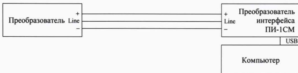
Рисунок 7 – Схема подключения преобразователей модификации ДТР-1-СМ, ДТР-2-СМ, ДТР-2Р-СМ.
