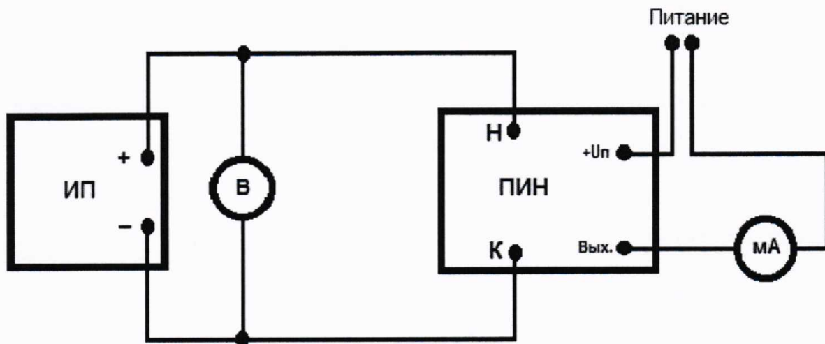
Рисунок 3 – Схема измерений при определении погрешности преобразования напряжения постоянного тока для преобразователей, ПИН-***-У-4/20-ДХ
