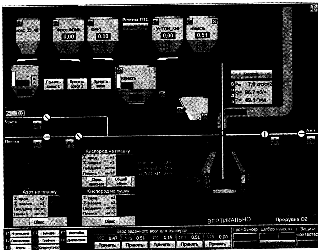
Рисунок 1- Отображение значений технологических параметров на экранной форме «Мнемосхема»
