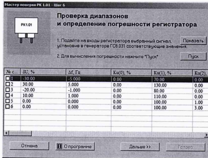
Рисунок А.3.7 - Вид окна «Проверка диапазонов и определение погрешности регистратора» программы «Мастер поверки РК1.01»
