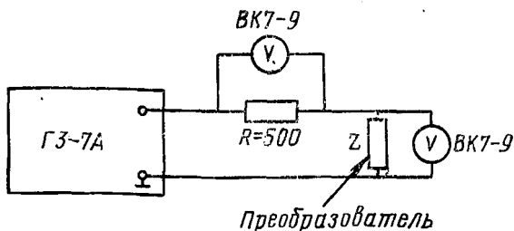
Схема для определения резонансной частоты преобразователя
