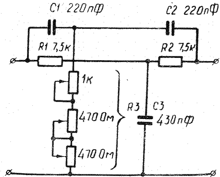
Рис. 4. Схема электрическая принципиальная RC-фильтра
