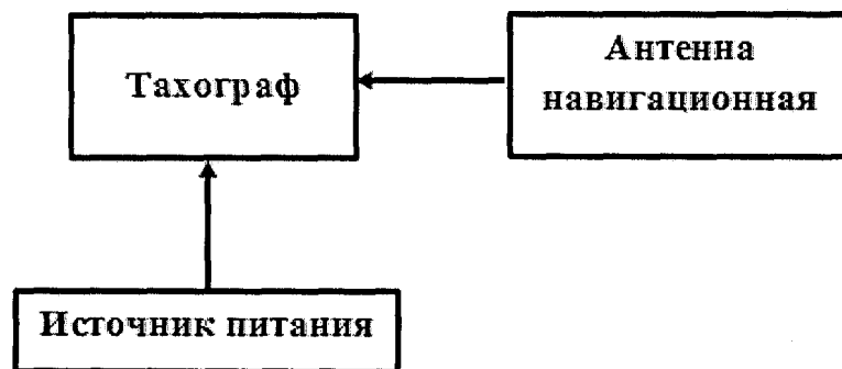
Рисунок 1 – Схема проведения измерений при проверке работоспособности
