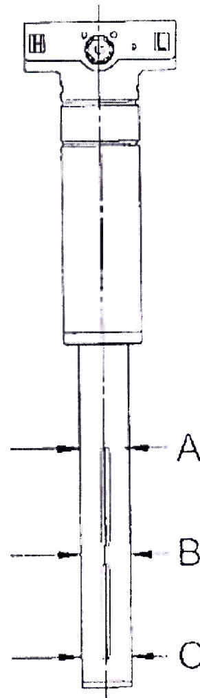
Рисунок А.1. – Схема измерений линейных размеров ОНТ
