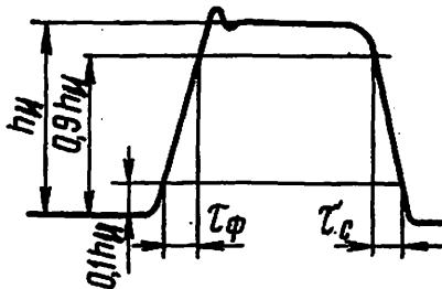
Рис. 12. Осциллограмма прямоугольного импульса сигнала калибровки коэффициента отклонения канала вертикального отклонения осциллографов:
