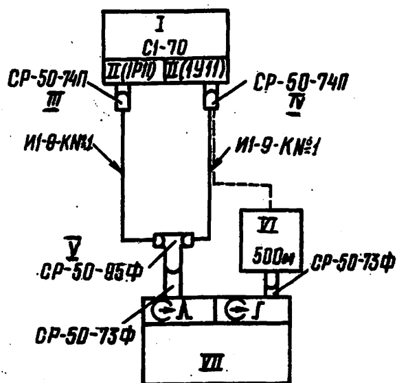
Рис. 14. Схема соединения приборов для определения установки задержки:
