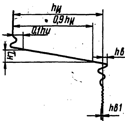
Рис. 13. Осциллограмма времени нарастания, величины выброса и неравномерности вершины переходной характеристики:
