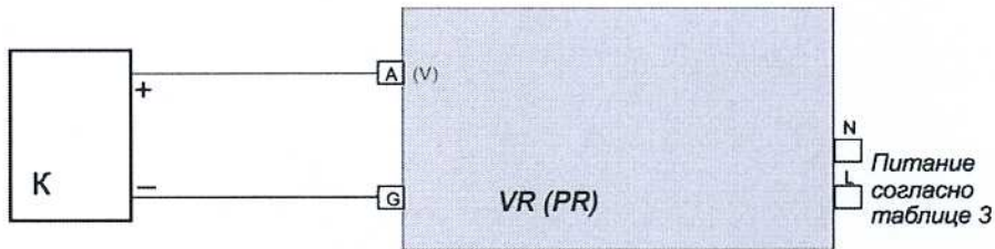
Рисунок А.1 – Схема подключения приборов при определении основной погрешности регистраторов с входными сигналами постоянного тока
