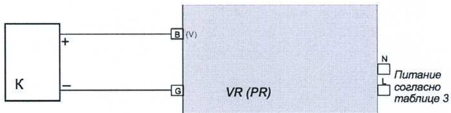
Рисунок А.2 – Схема подключения приборов при определении основной погрешности регистраторов с входными сигналами напряжения (В) постоянного тока
