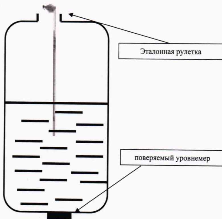
Рисунок Б.1 - Проверка уровнемера без демонтажа по месту эксплуатации
