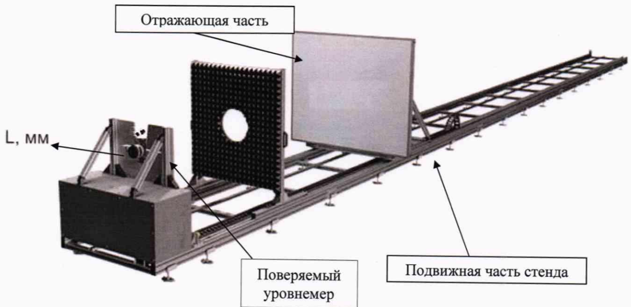
Рисунок А.1 - Проверка уровнемера на поверочной установке с непосредственным изменением уровня жидкости
