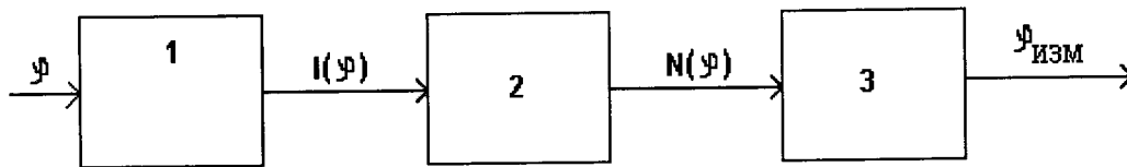
Рисунок 9. Функциональная схема модуля измерений относительной влажности МИВ
