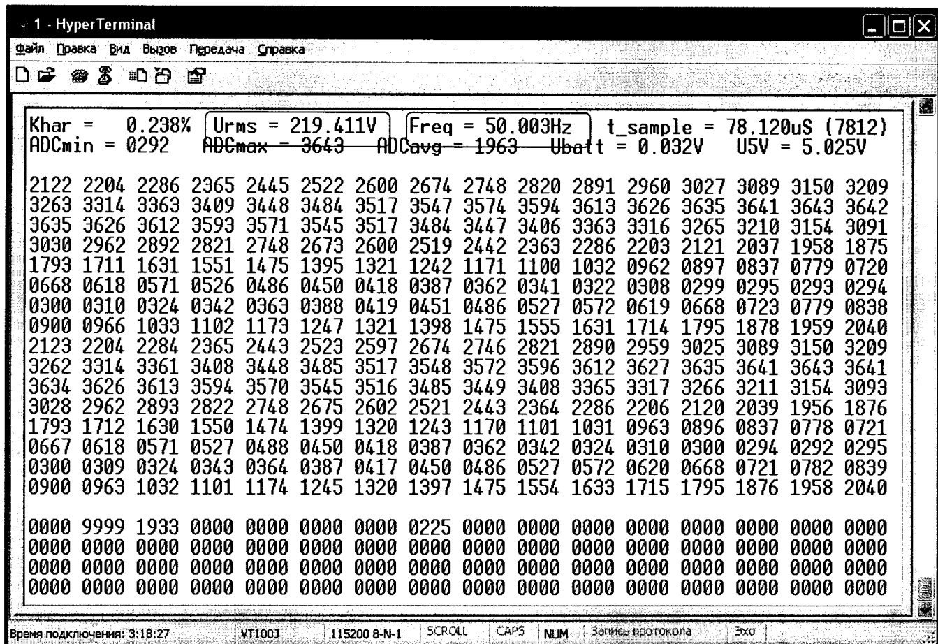
Рисунок 7 – Окно измерений ADC ПИК-СТ
