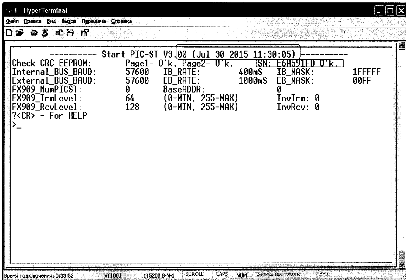
Рисунок 5 – Командное окно ПИК-СТ
