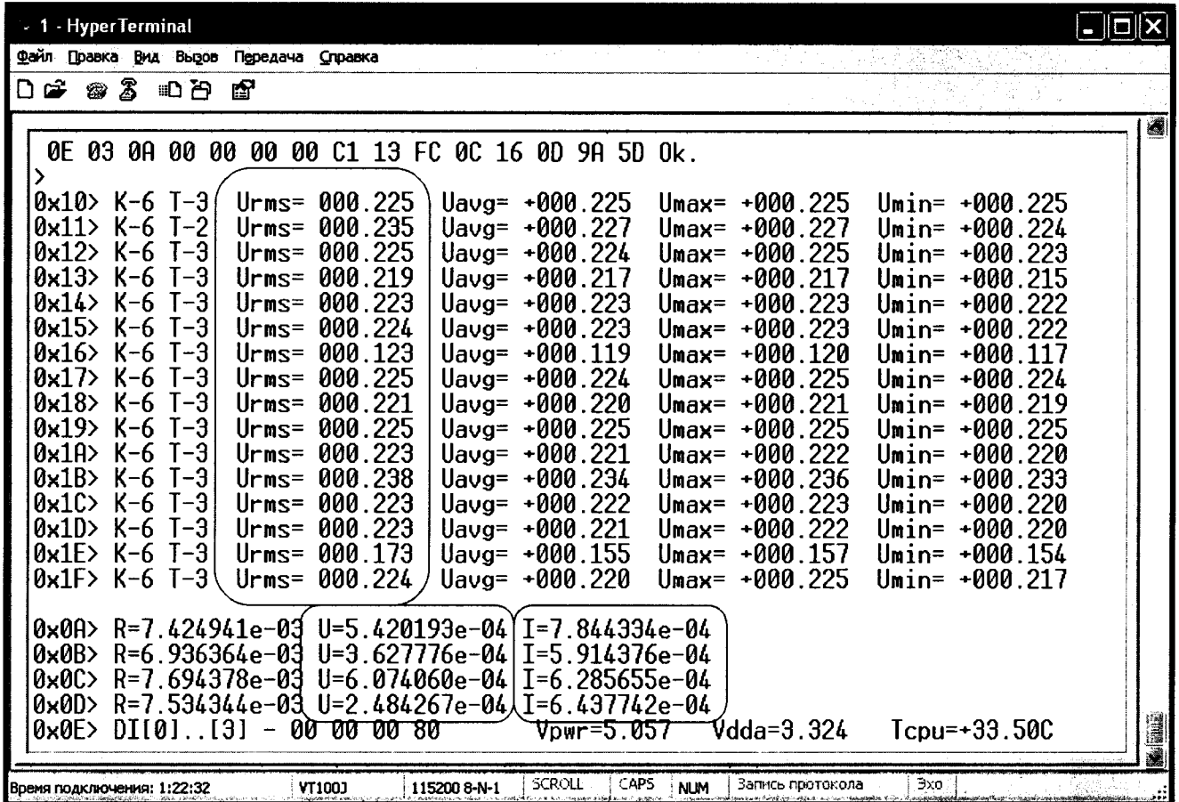
Рисунок 6 – Окно измерений ПИК-СТ
