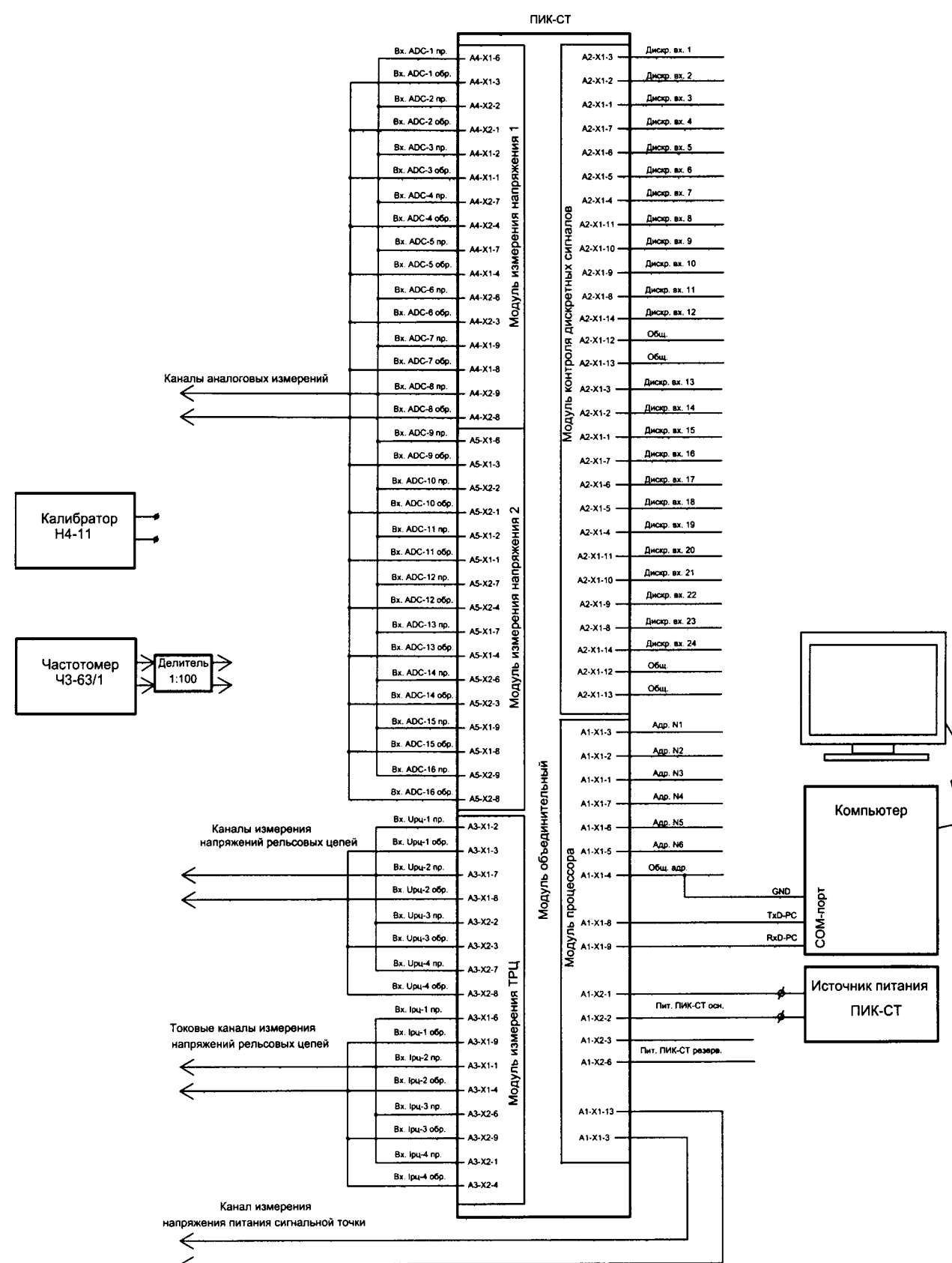
Рисунок 1 – Схема проведения поверки
