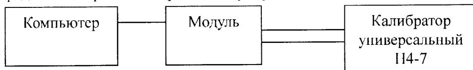
Рисунок 2 – Схема соединений
