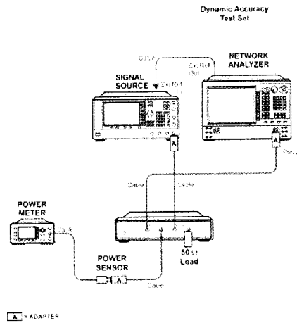
Рисунок 2 – Структурная схема измерения P_{mT} при определении нелинейности приемника измерителя коэффициента шума
