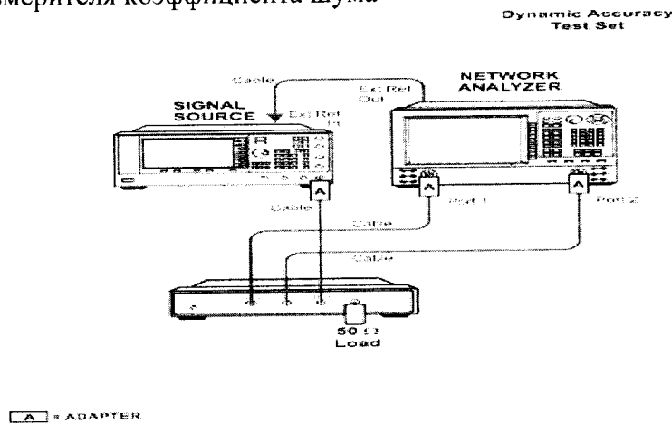
Рисунок 3 – Структурная схема измерения P_{mR} при определении нелинейности приемника измерителя коэффициента шума
