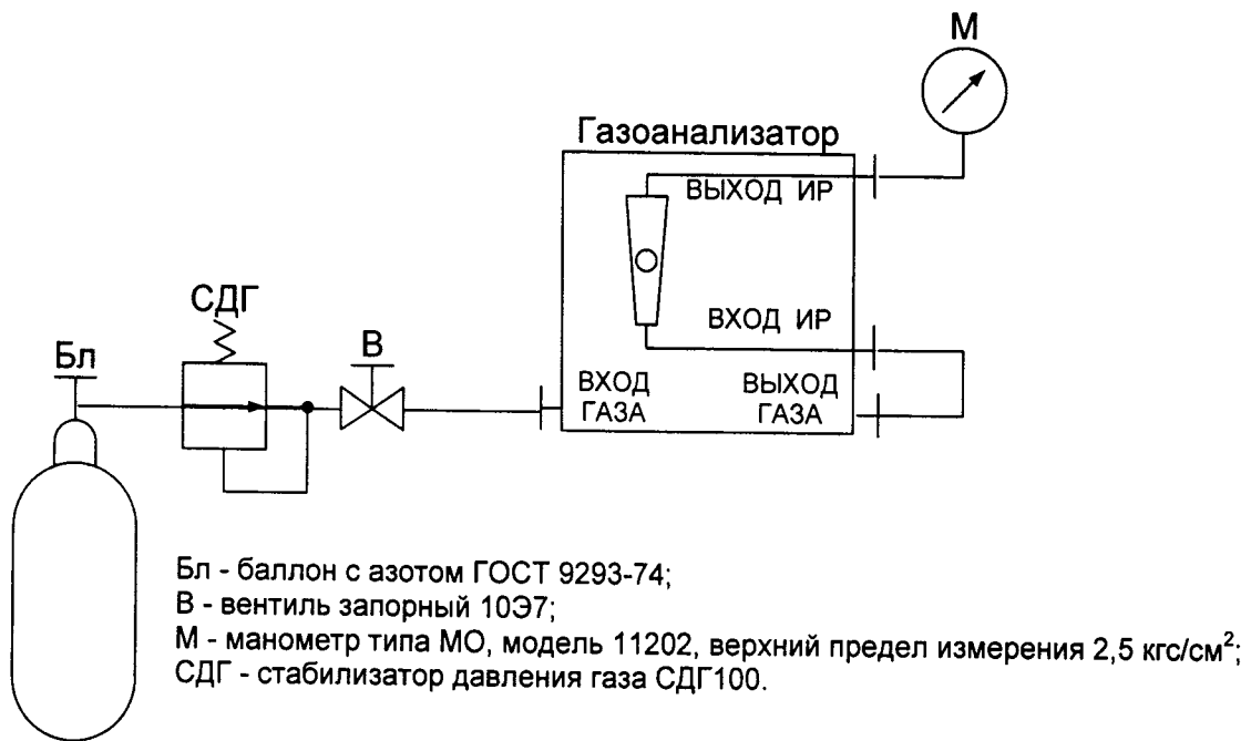
Рисунок Б.1 - Пневматическая схема проверки герметичности газового канала газоанализатора и газового канала индикатора расхода газа
