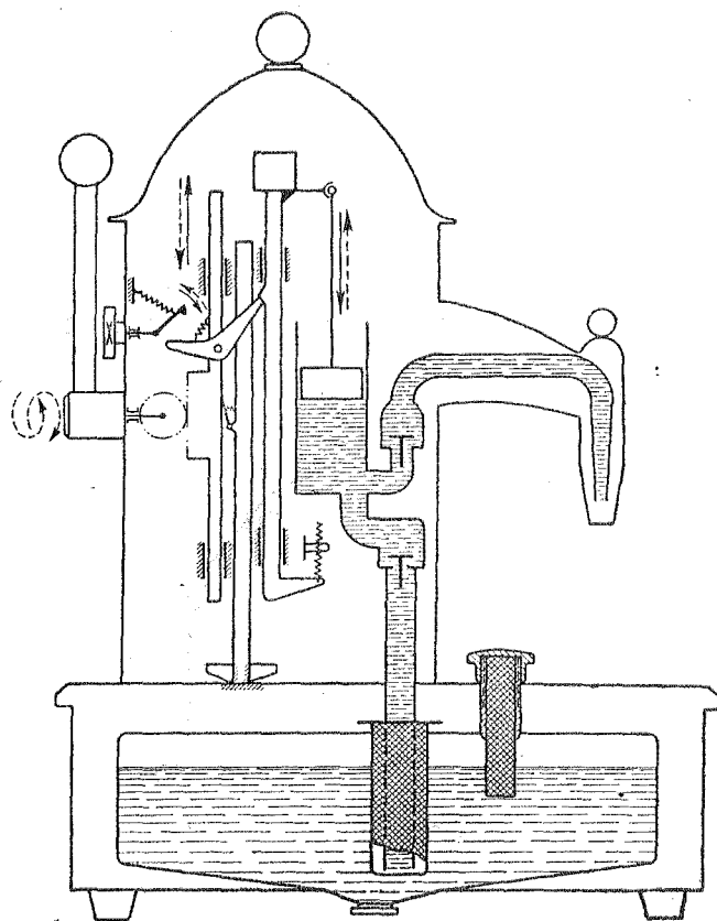
Схема дозатора водки, типа ДН
