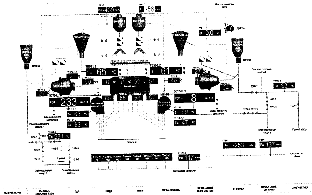
Рисунок 1 - Отображение значений технологических параметров на экранной форме «Пыль»
