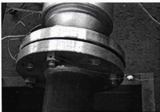
Рисунок 1 - Пломба поверителя, препятствующая демонтажу счетчика-расходомера массового
