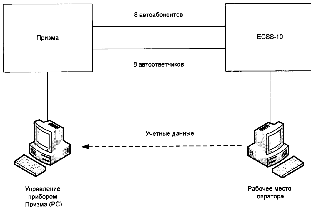
Рисунок 1- Схема поверки
