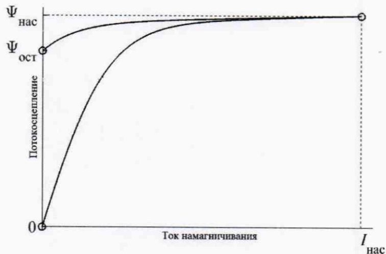
Рисунок 3 – Характерный вид зависимости потокосцепления от тока намагничивания в опыте по определению коэффициента остаточной намагниченности
