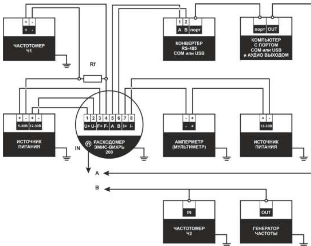
Рисунок П.1 – Схема подключения расходомеров при определении метрологических характеристик имитационным способом
