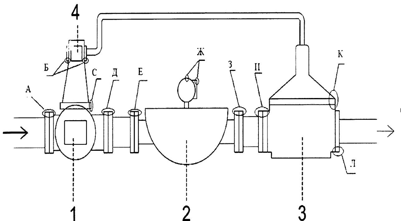
Рисунок 1 – Гидравлическая схема установок «Cogio T» с точками пломбирования
