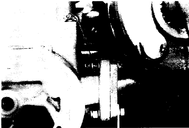
Рисунок 2 – Места пломбировки элементов гидравлического модуля установок «Согіо Т»
