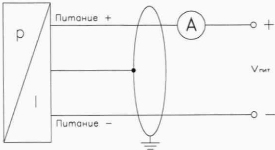
2-х пров. (вых. сигнал - ток)
