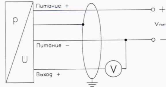
3-х пров. (вых. сигнал - напряжение)
