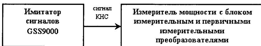
Рисунок 3 – Схема измерений для определения погрешности установки уровня мощности выходных сигналов
