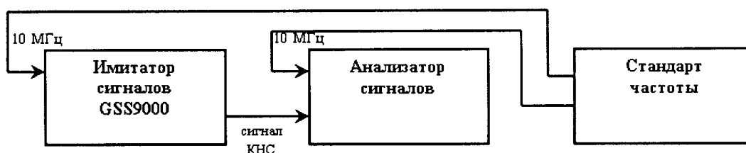
Рисунок 2 – Схема измерений для определения уровня гармонических составляющих
