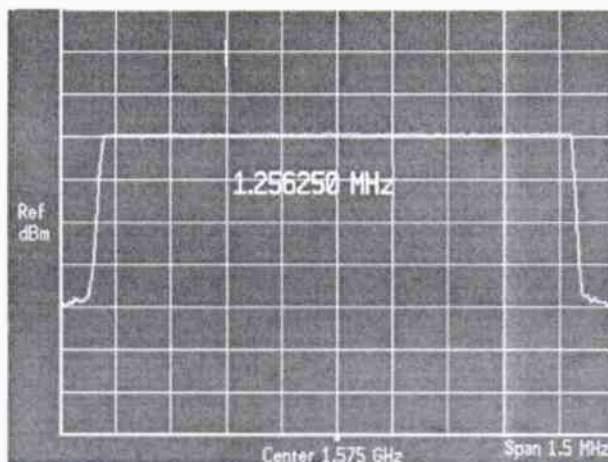
Рисунок 8 – Смещение несущей частоты навигационного сигнала относительно номинального значения 1,57542 ГГц
