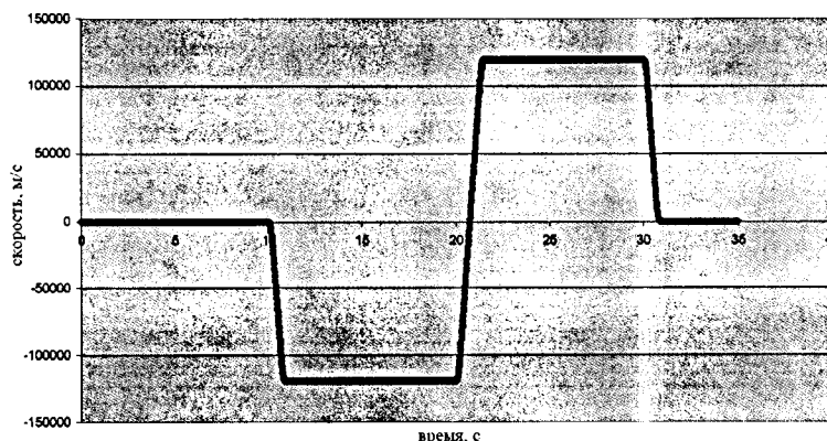
Рисунок 7 – График изменения скорости объекта типа «самолет»
