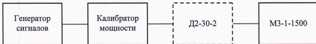
Рисунок 1 – Схема определения относительной погрешности измерений мощности
