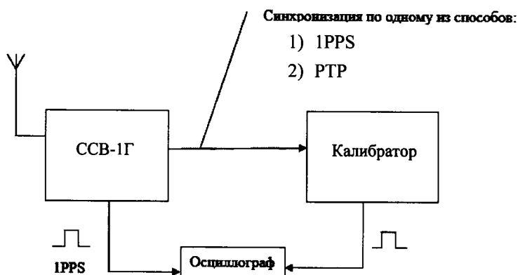
Рисунок 3 – Проверка пределов допускаемой погрешности измерения текущего времени.
