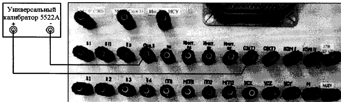
Рисунок 145 – Схема подключения для проверки напряжения по цепи «С3т»
