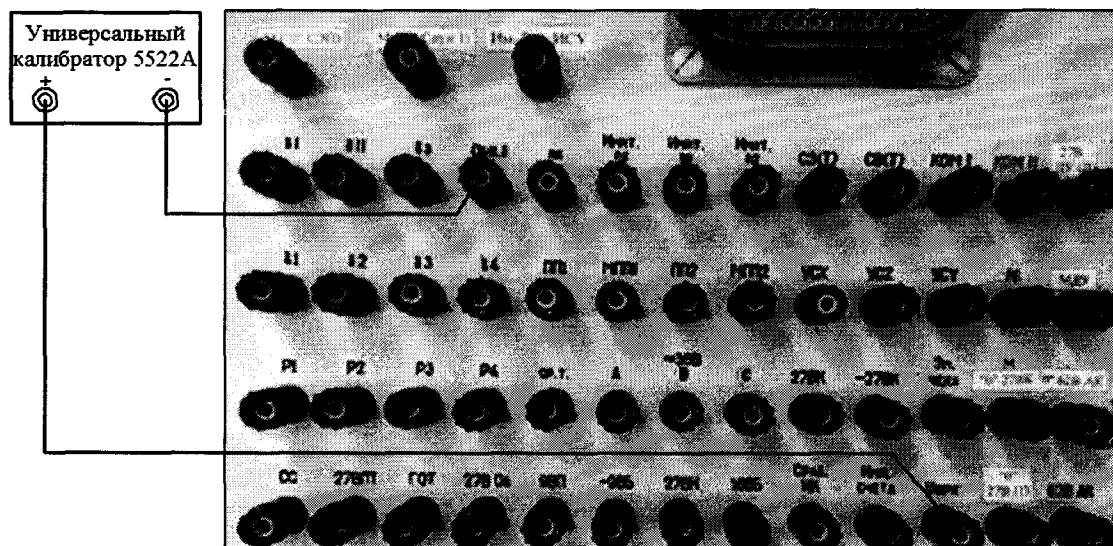
Рисунок 147 – Схема подключения для проверки напряжения по цепи «Ушрк»
