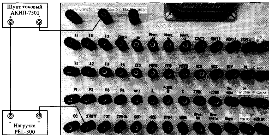
Рисунок 133 – Схема измерений силы постоянного тока по цепи «27 В ПТ»
