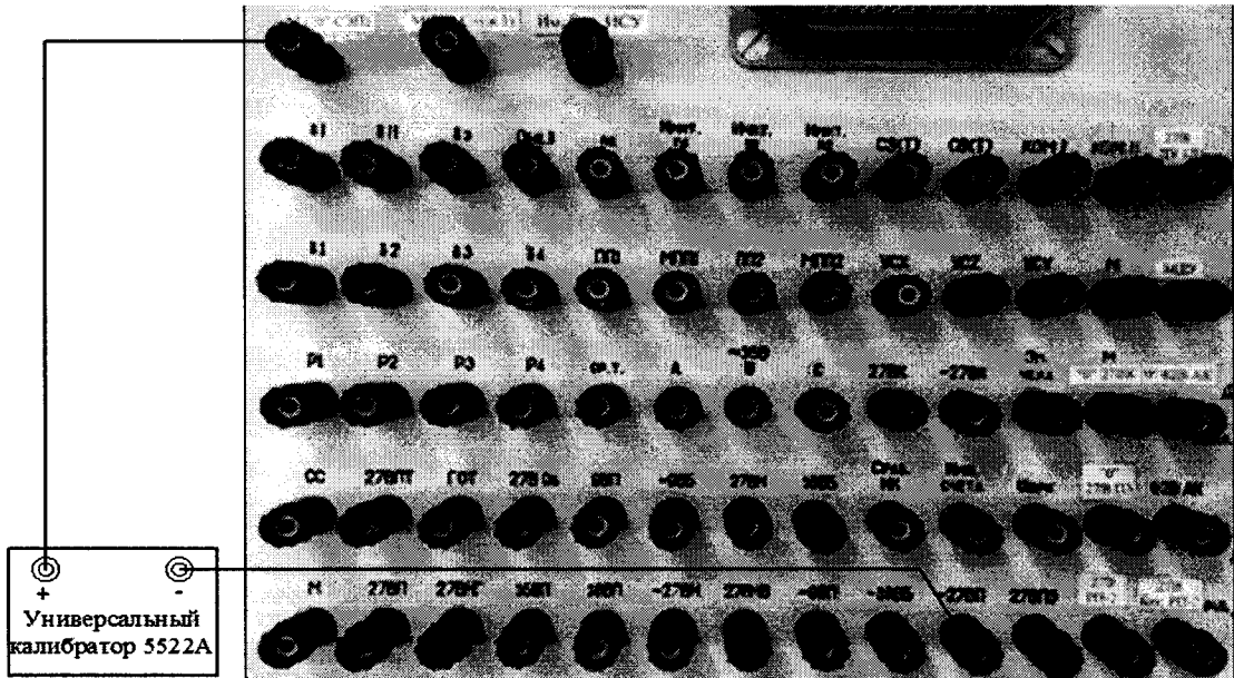
Рисунок 54 – Схема подключения для проверки напряжения по цепи «- 27 В П»
