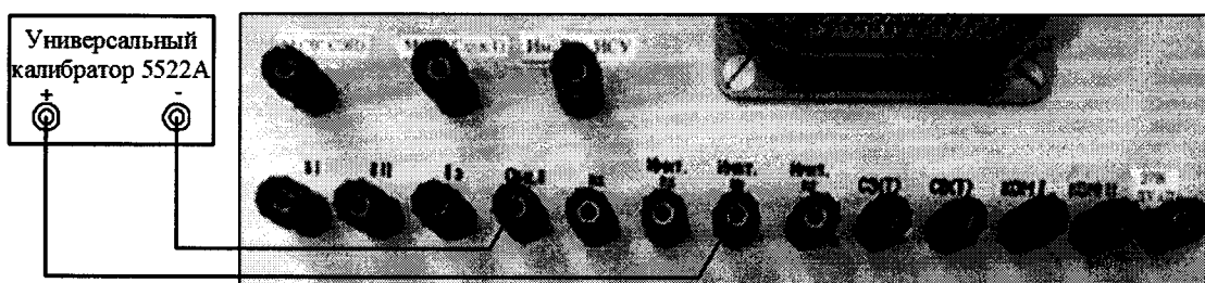
Рисунок 137 – Схема подключения для проверки напряжения по цепи «Имит пу»
