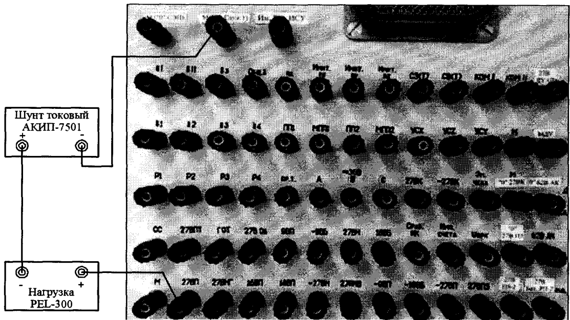
Рисунок 118 – Схема измерений силы постоянного тока по цепи «27 В П»
