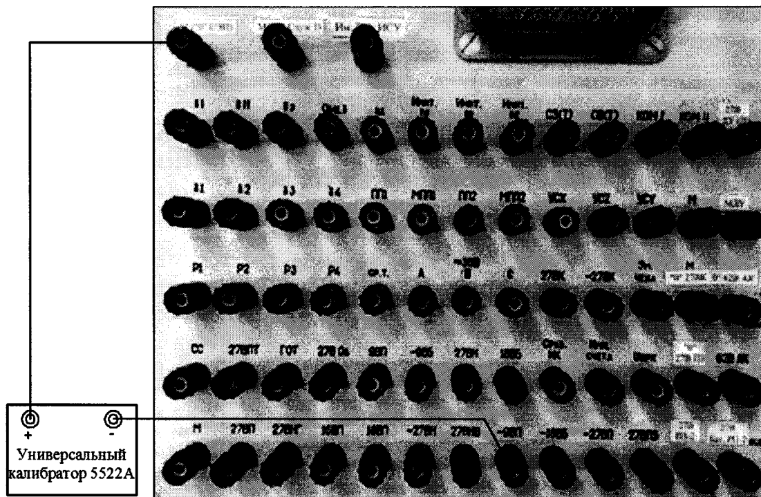
Рисунок 36 – Схема подключения для проверки напряжения по цепи «- 9 В П»
