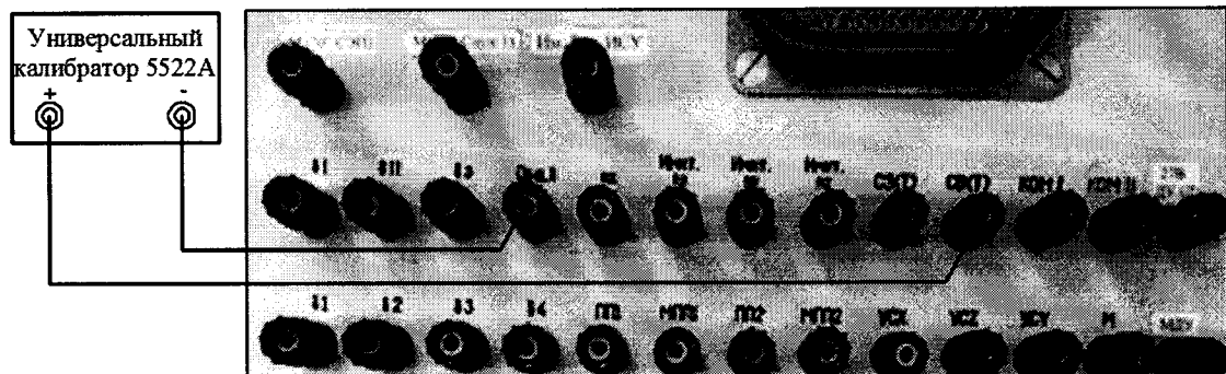
Рисунок 143 – Схема подключения для проверки напряжения по цепи «СВт»
