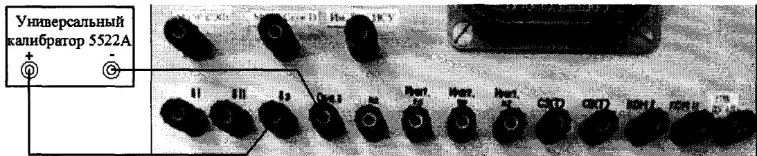
Рисунок 167 – Схема подключения для проверки напряжения по цепи «delta»
