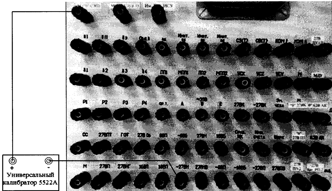
Рисунок 57 – Схема подключения для проверки напряжения по цепи «- 27 В Н»
