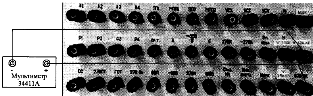
Рисунок 84 – Схема подключения для проверки напряжения по цепи «62 В АК»
