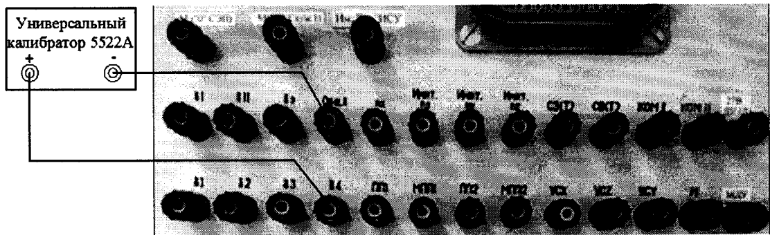
Рисунок 175 – Схема подключения для проверки напряжения по цепи «delta 5»
