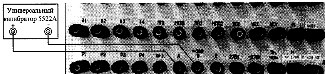
Рисунок 177 – Схема подключения калибратора между фазами «А» и «В»
