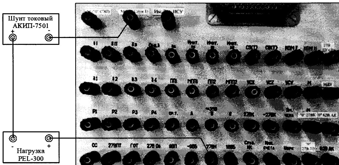
Рисунок 122 – Схема измерений силы постоянного тока по цепи «27 В Н»
