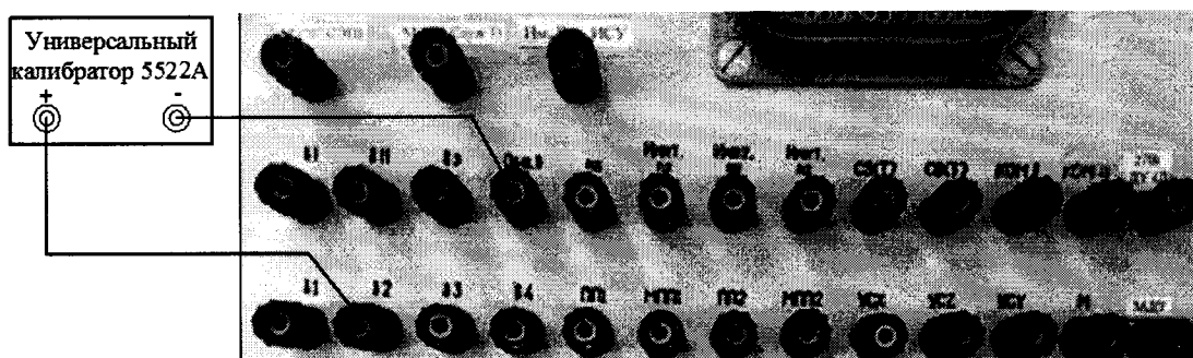
Рисунок 171 – Схема подключения для поверки напряжения по цепи « \delta 2 »
