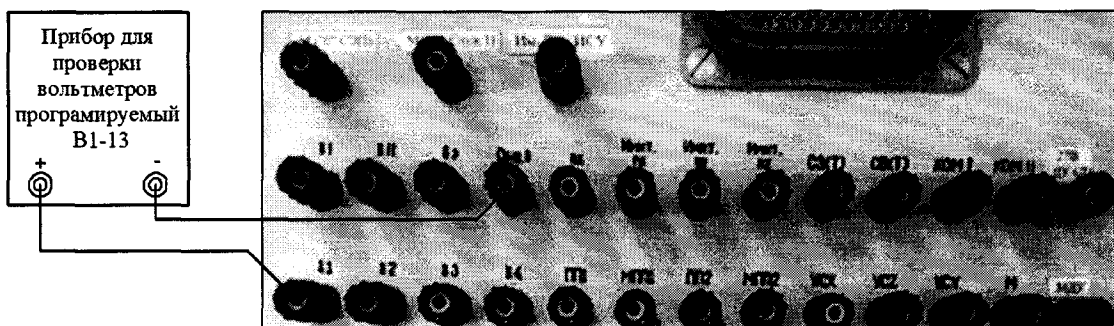
Рисунок 169 – Схема подключения для проверки напряжения по цепи «delta I»
