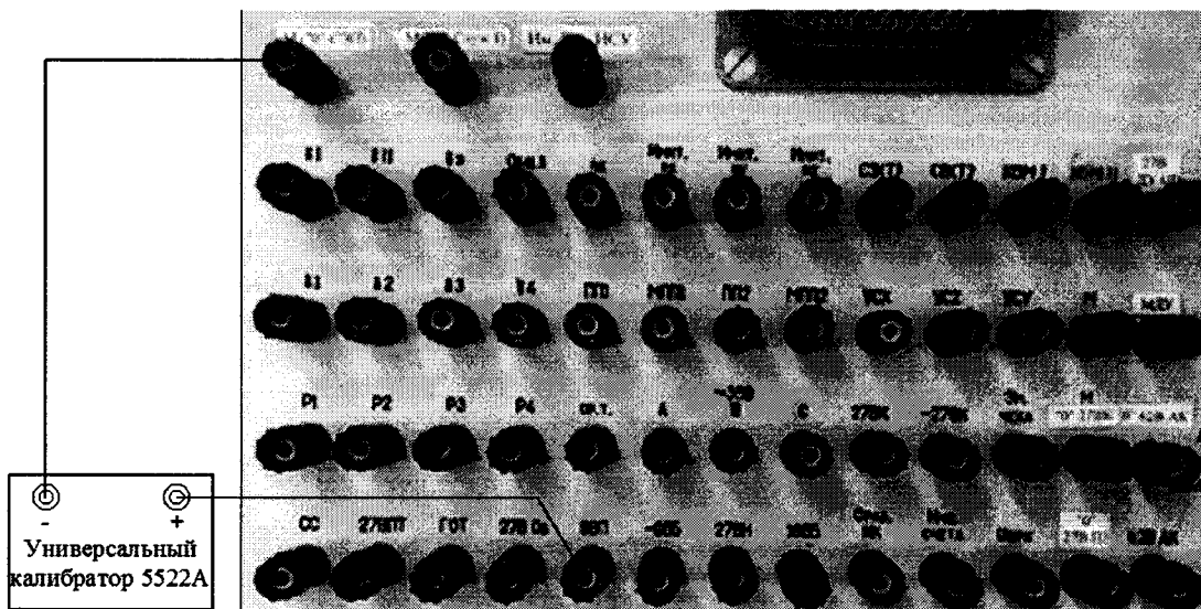
Рисунок 40 – Схема подключения для поверки напряжения по цепи «9 В П (хх)»
