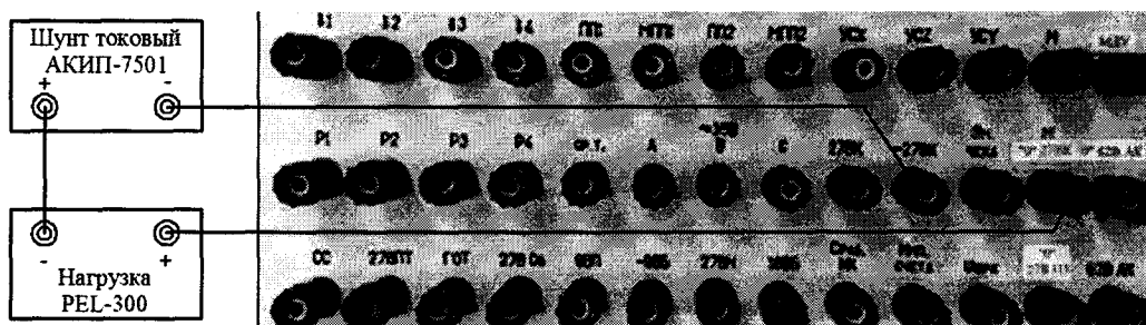
Рисунок 116 – Схема измерений силы постоянного тока по цепи «- 27 В К»
