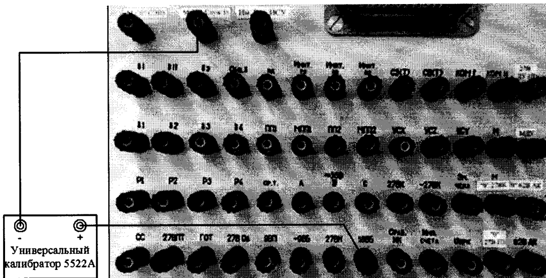
Рисунок 49 – Схема подключения для проверки напряжения по цепи «18 В Б»
