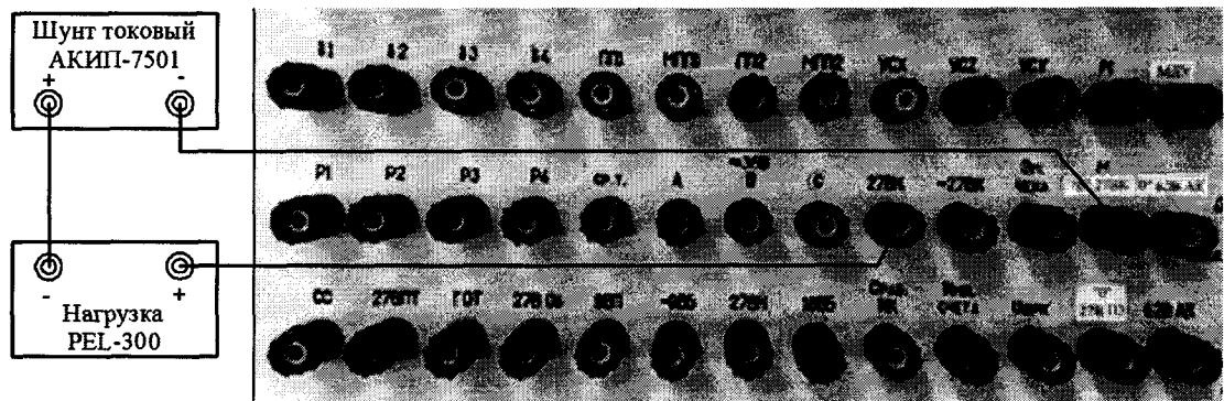
Рисунок 114 – Схема измерений силы постоянного тока по цепи «27 В К»
