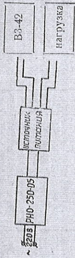
Рис. 5. Структурная схема измерения пульсации выходного напряжения
