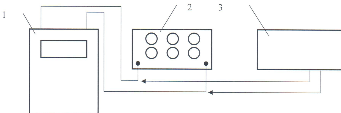
Рисунок 1 – Схема соединений при поверке прибора «Вымпел» в режиме измерений активного сопротивления.
