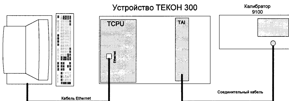
Рисунок 4 – Схема для проверки пределов допускаемой основной абсолютной погрешности измерений среднеквадратических значений силы переменного тока при I_{\text{НОМ}}=1 А
