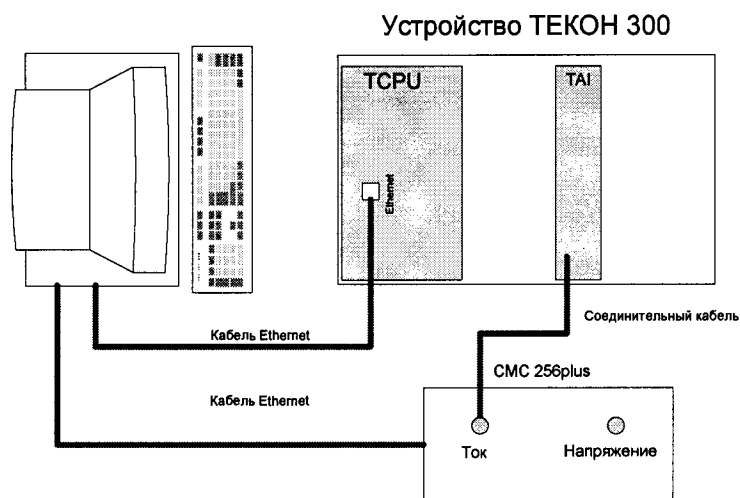
Рисунок 5 – Схема для проверки пределов допускаемой основной абсолютной погрешности измерений среднеквадратических значений силы переменного тока при I_{\text{НОМ}}=5 \text{ А}
