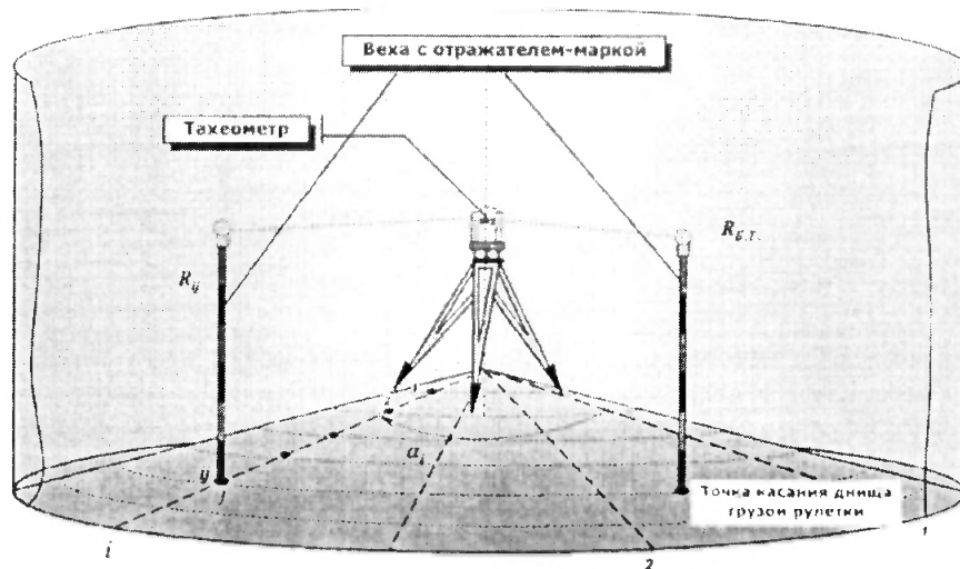
Рисунок А.5 Определение параметров дна резервуара
