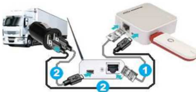
Рисунок 2.8 – Подключение менеджера WST-EMT к Интернету через портативный беспроводной маршрутизатор с подключённым к нему GSM-модемом с использованием автомобильного адаптера для прикуривателя
