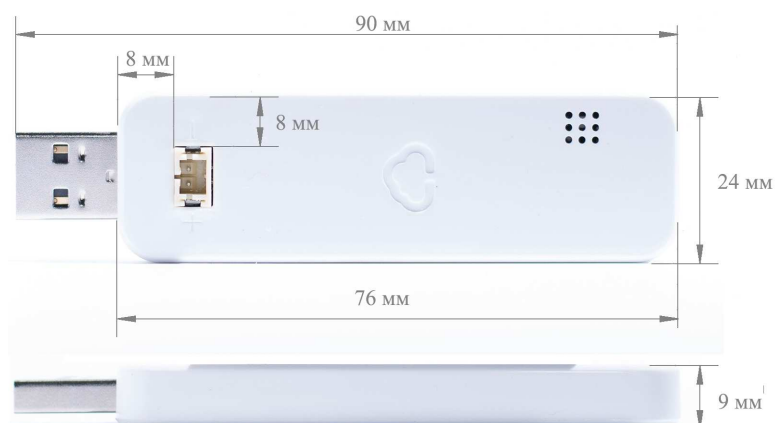
Рисунок 1.3 - Внешний вид и размеры тегов комплекса WSTR
