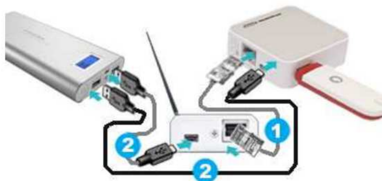
Рисунок 2.7 – Подключение менеджера WST-EMT к Интернету через портативный беспроводной маршрутизатор с подключённым к нему GSM-модемом
