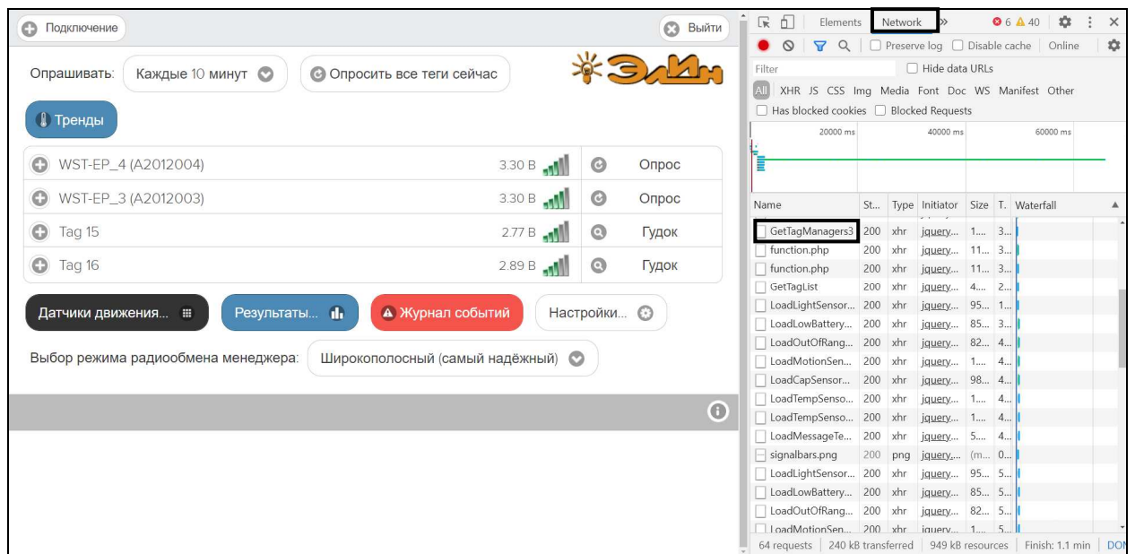
Рисунок 3.4 – Внешний вид страницы разводящего окна веб-сервиса WST_WebUI и отладочной консоли браузера Google Chrome. Вкладка «Network» и пункт {GetTagManagers#} выделены чёрными рамками.
