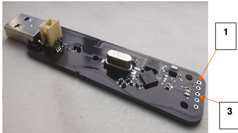
Рисунок 2.87 – Контакты на плате тега, которые необходимо замкнуть проводником для исполнения операции аппаратной очистки флэш-памяти тега
