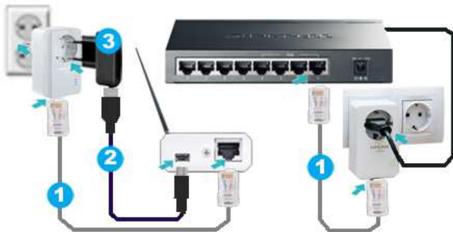
Рисунок 2.2 – Подключение менеджера WST-EMT через репитер к проводному Интернету
