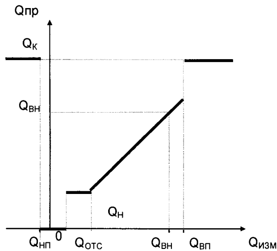
Рисунок 4.2 – Преобразование измеренных значений объемного расхода
