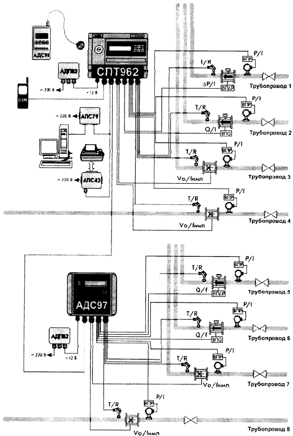
Рисунок 2.1 – Система с открытым водоразбором
