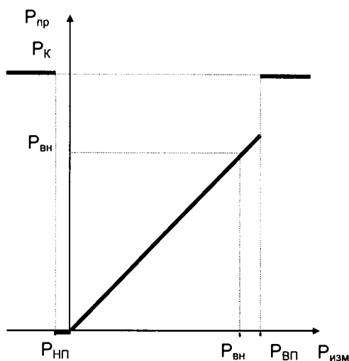
Рисунок 4.5 Преобразование измеренных значений давления
