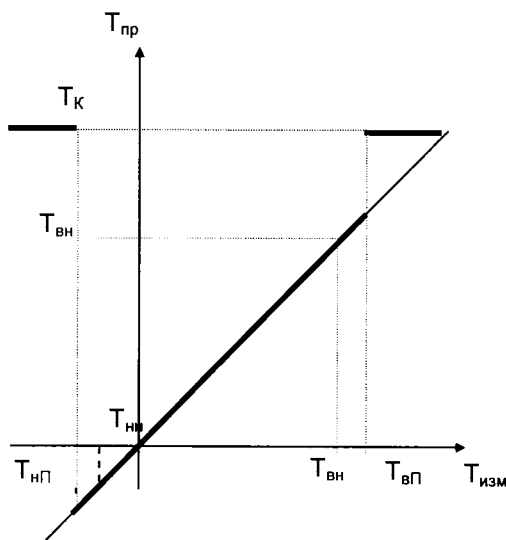
Рисунок 4.4 Преобразование измеренных значений температуры
