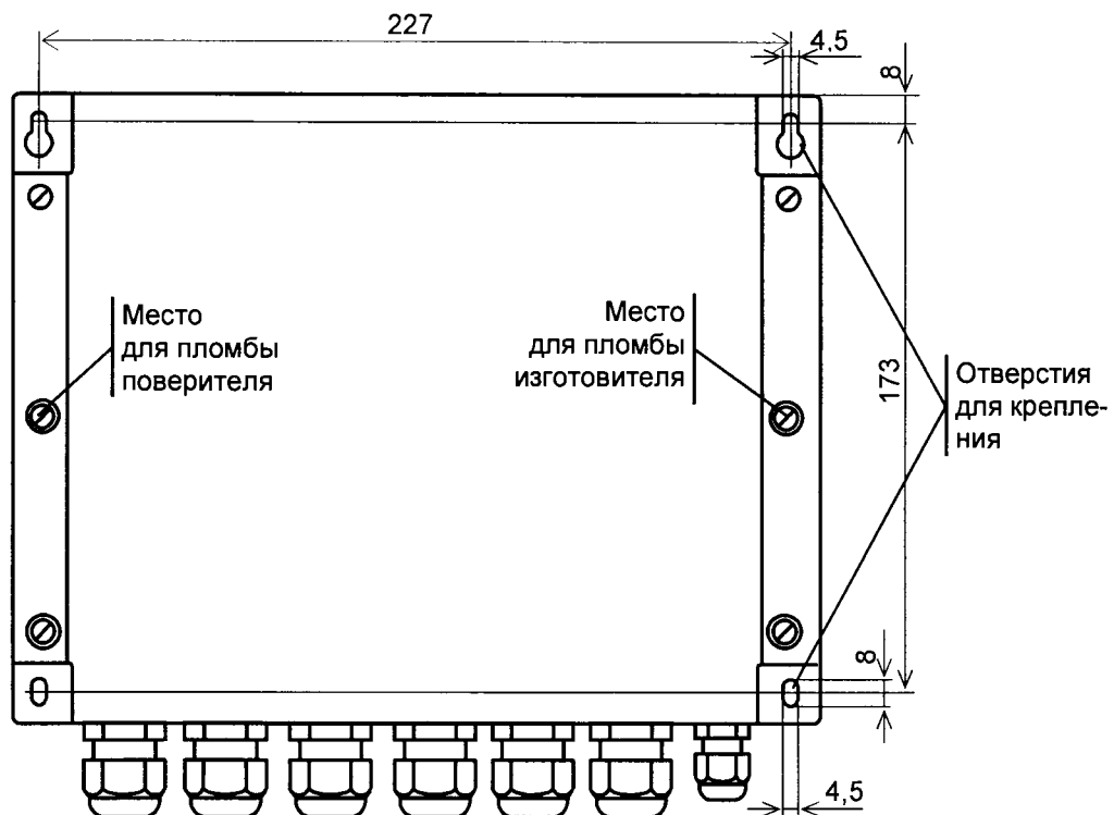
Рисунок 3.3 – Вид сзади
