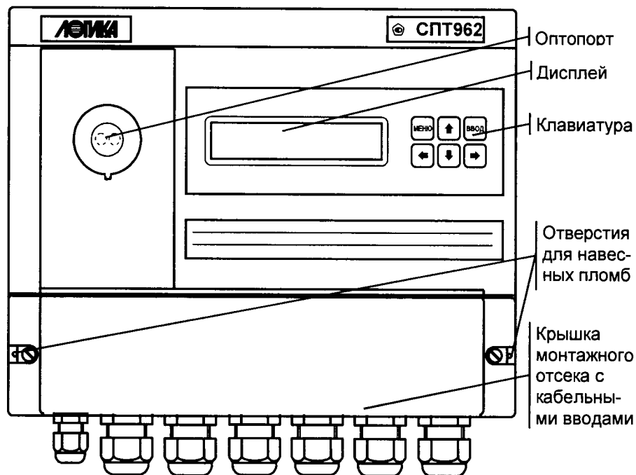
Рисунок 3.1 – Вид спереди
