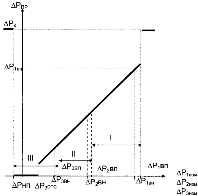
Рисунок 4.6 – Преобразование значений перепада давления, измеренных тремя датчиками
