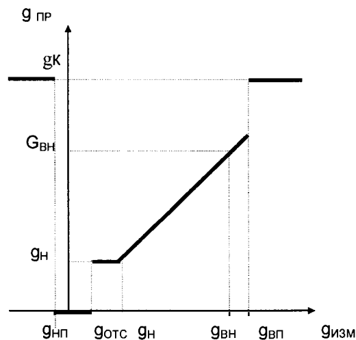
Рисунок 4.3 – Преобразование измеренных значений массового расхода
