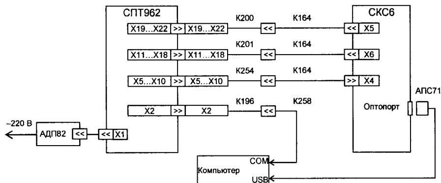
Рисунок 11.1 – Схема проверки
