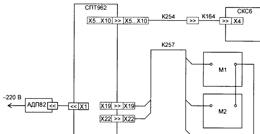
Рисунок 11.2 – Схема проверки. М1, М2 – магазин сопротивлений Р4831
