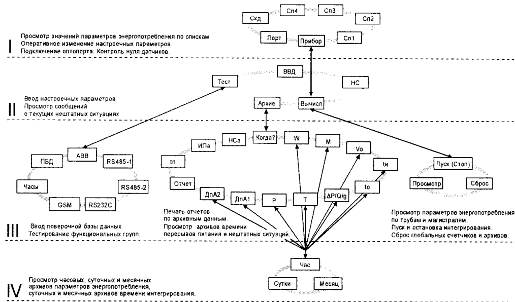
Рисунок 6.1 – Структура меню
