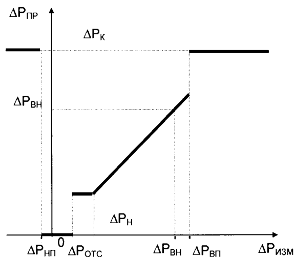
Рисунок 4.1 – Преобразование измеренных значений перепада давления
