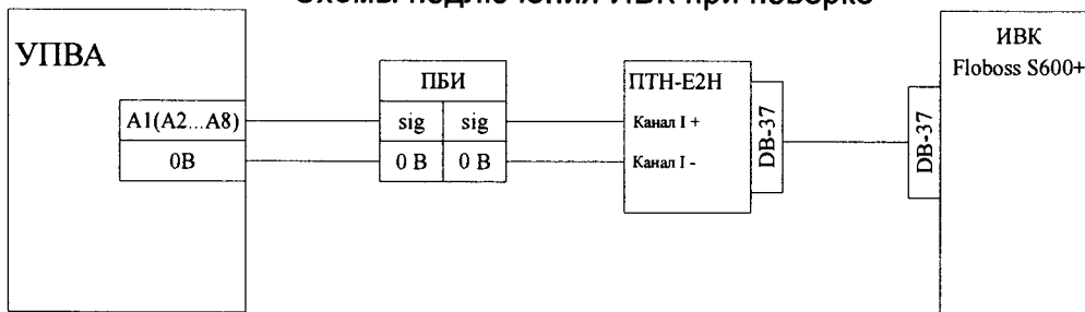
Рисунок Б.1. Схема подключения средств поверки при определении погрешности преобразования входных аналоговых сигналов в значения физических величин, а также при проведении калибровки аналоговых каналов ИВК (ПБИ -пассивный барьер искробезопасный; ПТН-Е2Н – преобразователь измерительный постоянного тока)
