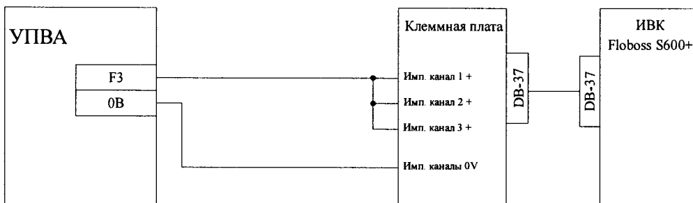
Рисунок Б.3. Схема подключения средств поверки при определении погрешности преобразования входных сигналов в значения объема и массы нефти
