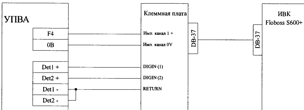
Рисунок Б.4. Схема подключения средств поверки при определении погрешности преобразования входных сигналов в значения преобразования массового ПР
