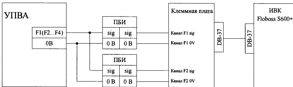
Рисунок Б.2. Схема подключения средств поверки при определении погрешности преобразования входных сигналов в значения плотности нефти
