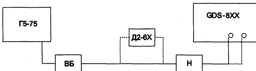
Н- нагрузка 50 Ом из комплекта Г5-75 ВБ - выносной блок генератора Г5-75
