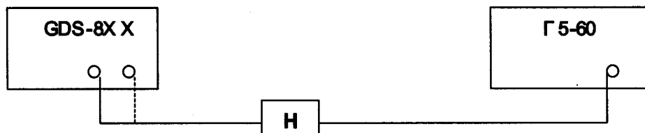
Н- нагрузка 50 Ом из комплекта Г5-75
