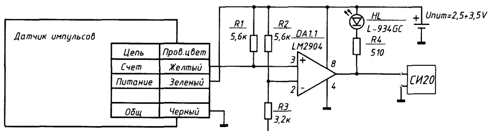
Рисунок 1 – Схема проверки счета импульсов
