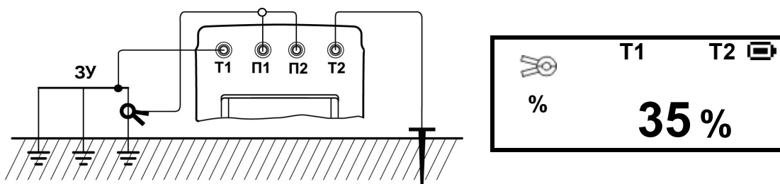
Рисунок 2.3.8 - Схема подключения и вид индикатора при определении процентного распределения токов
