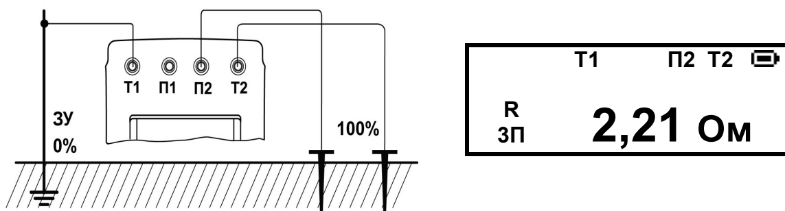
Рисунок 2.3.5 Схема измерения сопротивления заземления и вид индикатора при трёхпроводном методе измерения
