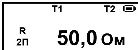
Рисунок 2.3.3.2 – Вид индикатора при двухпроводном методе измерения
