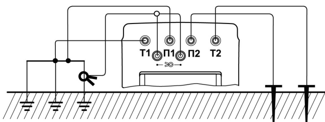
Рисунок 2.3.9 - Схема подключения и вид индикатора при измерении сопротивления единичного заземлителя
