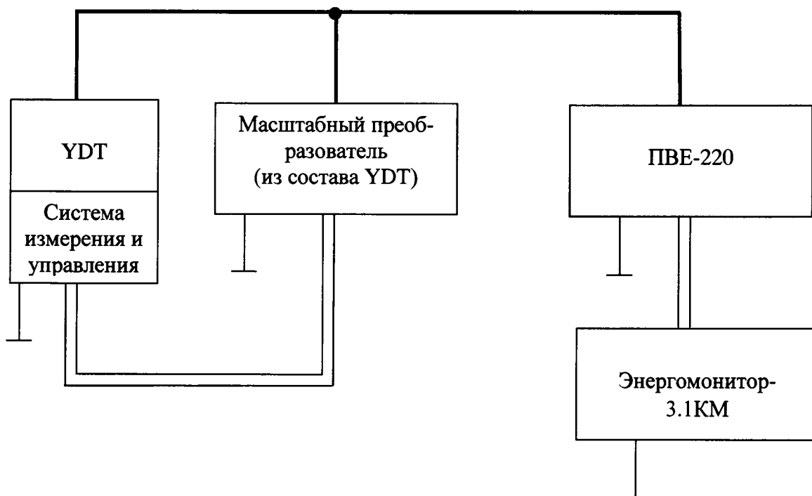
Рисунок 1 – Структурная схема проверки допускаемой относительной погрешности измерения и воспроизведения напряжения переменного тока
