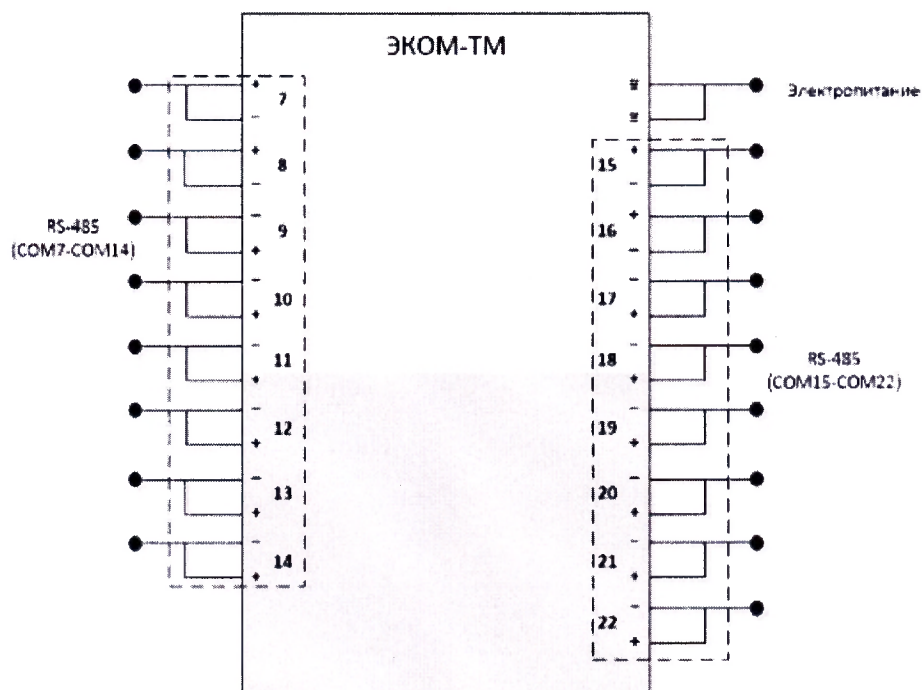
Рисунок 1 – Схема соединений для проверки электрического сопротивления изоляции и электрической прочности изоляции
