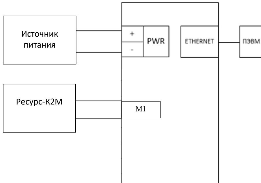
Рисунок 4 – Структурная схема определения погрешностей измерений фазного и междуфазного напряжения переменного тока, силы переменного тока, частоты переменного тока, электрического мощности и энергии, показателей качества электрической энергии
