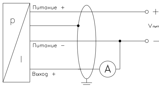
3-х пров. (вых. сигнал - ток)
