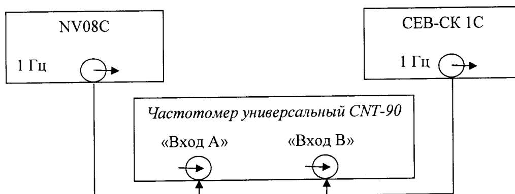
Рисунок 1 – Схема определения относительной погрешности по частоте
